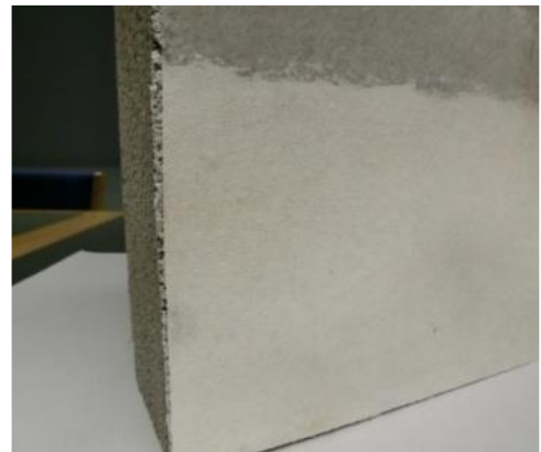
Abb: Wandmuster LAC 6 mit Dispersionspachtelmasse und eingearbeitetem Glasfasergewebe
